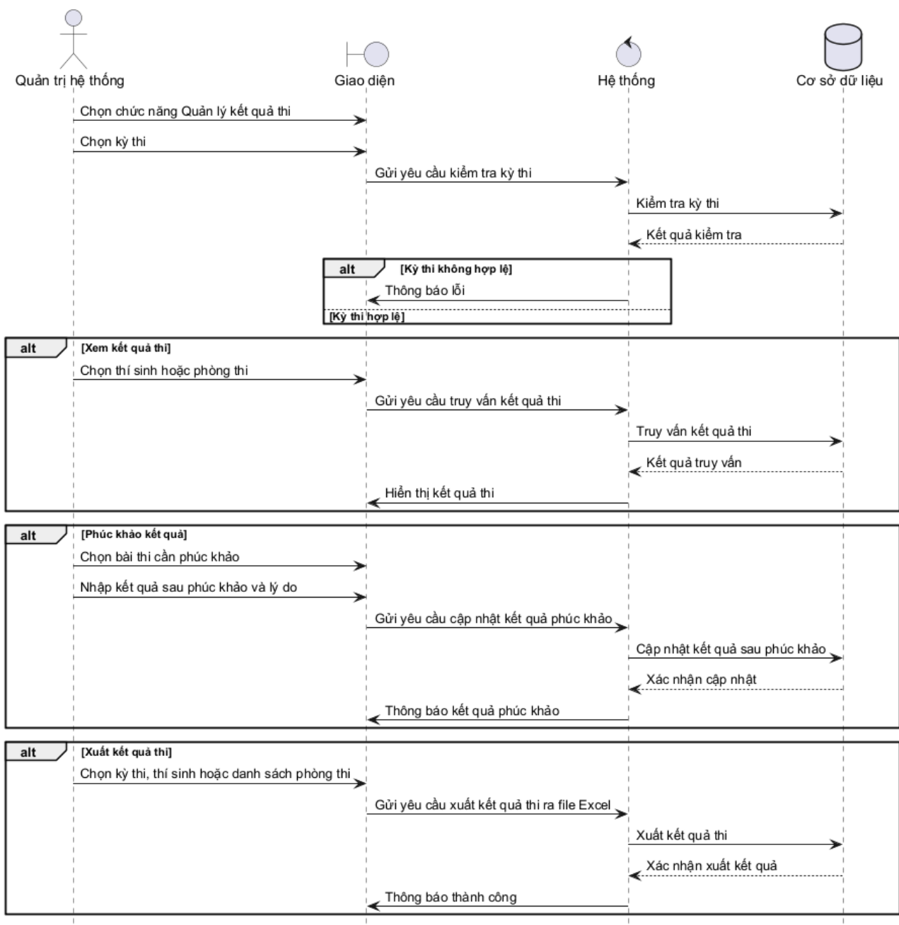
Hình 3.120: Sơ đồ tuần tự cho chức năng quản lý kết quả thi
