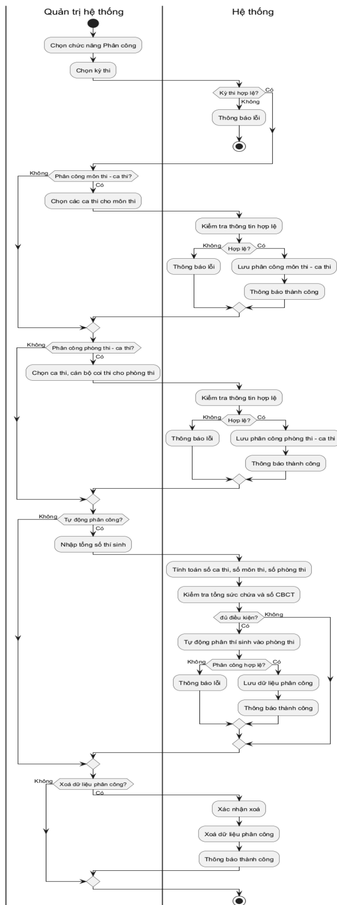
Hình 3.51: Sơ đồ hoạt động cho chức năng phân công
