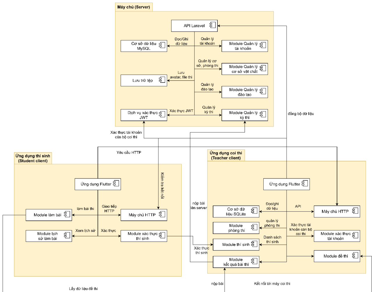
Hình 3.141: Sơ đồ thành phần
