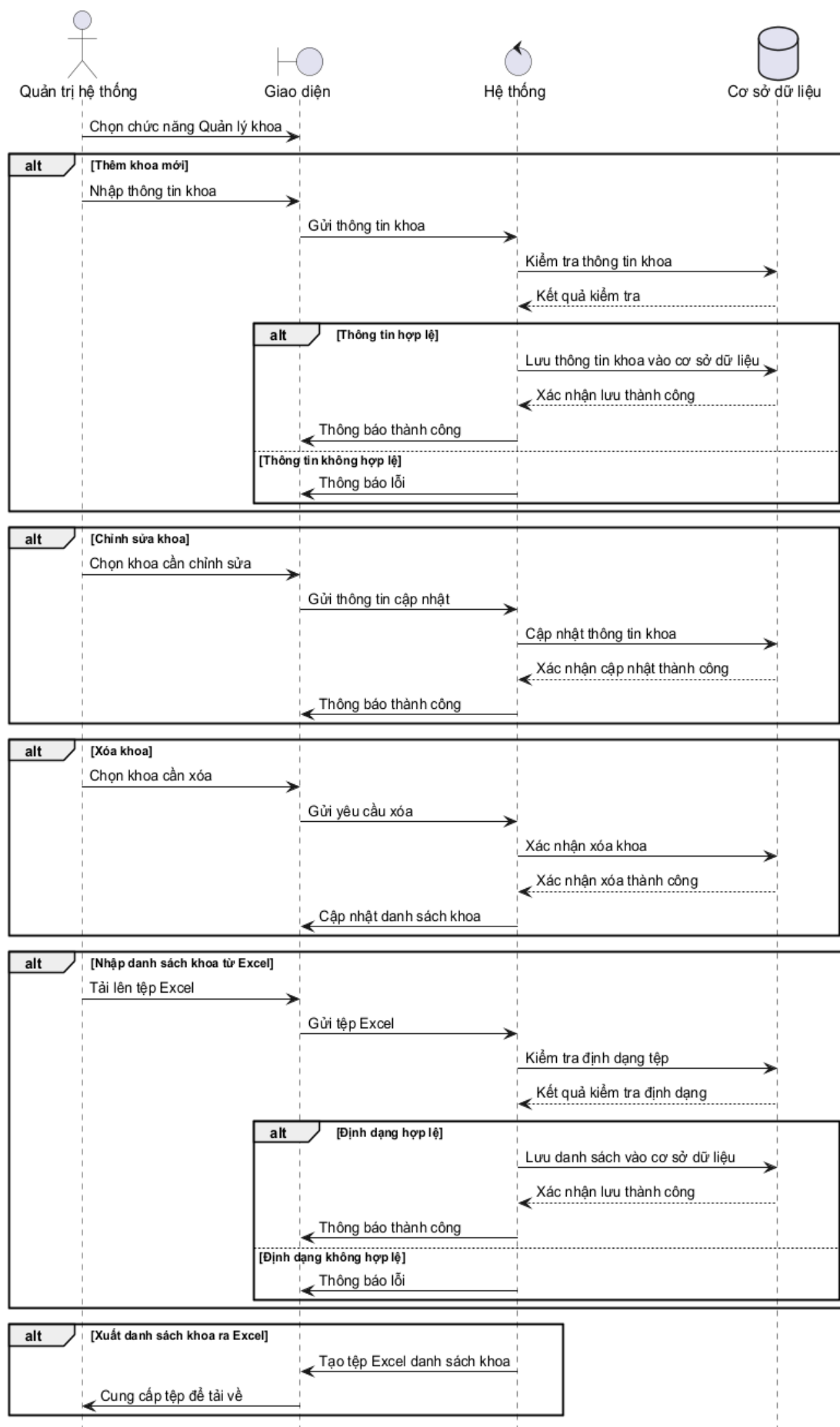
Hình 3.108: Sơ đồ tuần tự cho chức năng quản lý khoa
